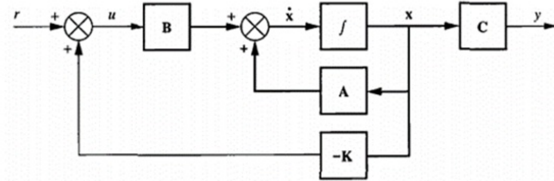
Gambar 4. Plant dengan kendali full state feedback
