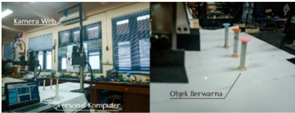
Sistem Keseluruhan Robot SCARA Serpent
